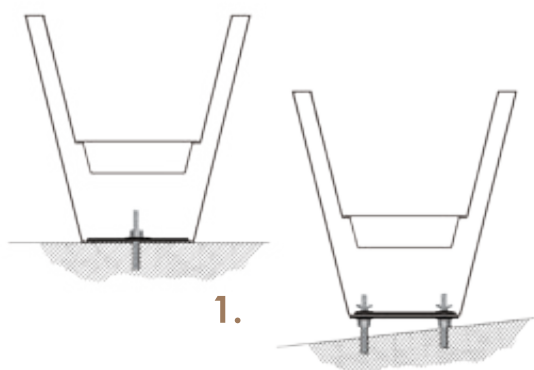
1 Ukotvení k zemi a ve svahu
